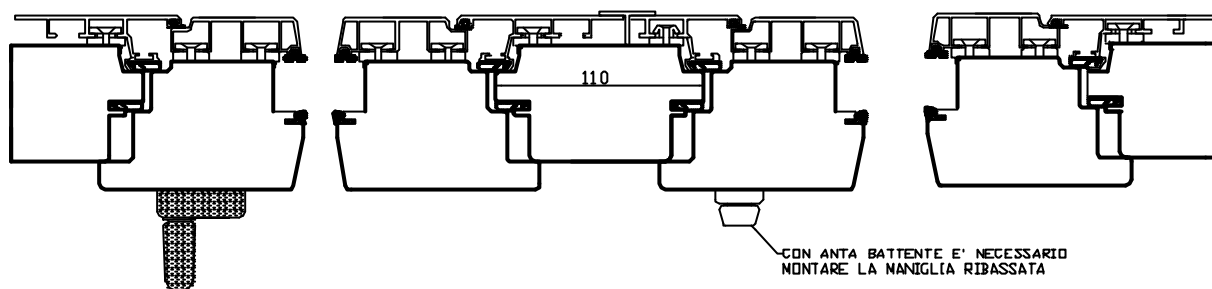
ANTA SCORREVOLE PIU' ANTA BATTENTE
