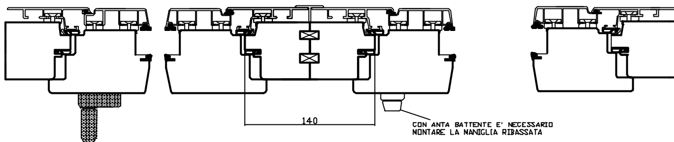
SEZIONE VERTICALE
