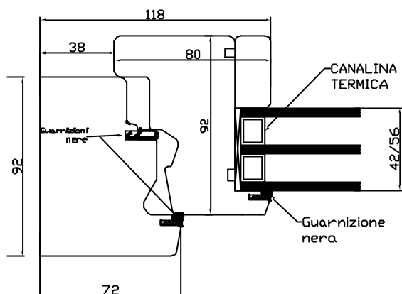
NODO LATERALE E SUPERIORE
