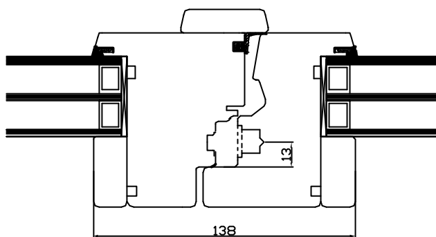
NODO INFERIORE CON TELAIO IN LEGNO RIDOTTO
