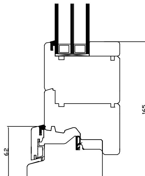
NODO INFERIORE CON TELAIO IN LEGNO RIDOTTO
