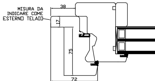
ALETTA STANDARD DA mm 20
